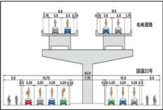
横断面図（イメージ）
